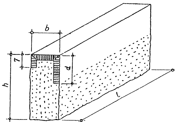
Rys. 1. Krawężnik uliczny odmiany UP, rodzaju A
