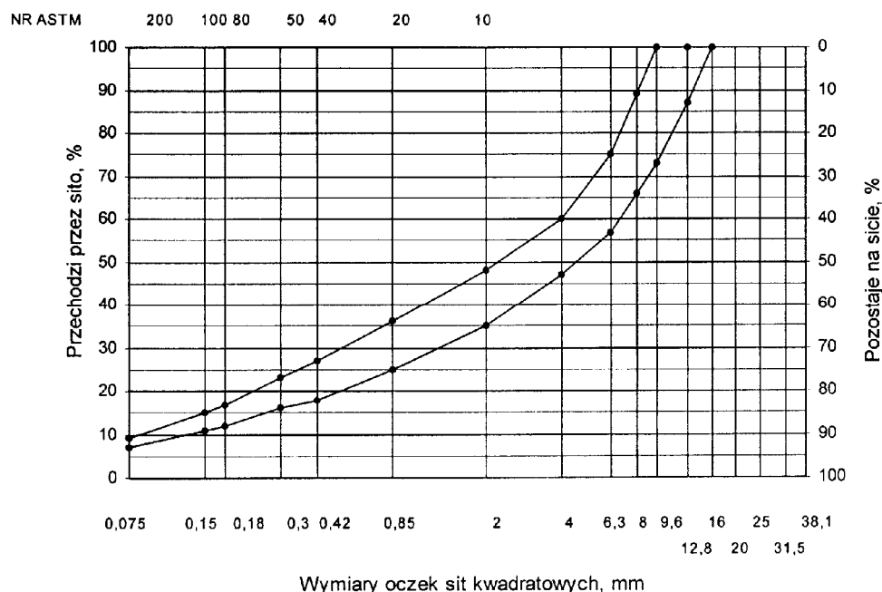
Rys. 3. Krzywe graniczne uziarnienia mieszanki mineralnej BA od 0 do 16 mm do warstwy ściernawej nawierzchni drogi o obciążeniu ruchem od KR3 do KR6
