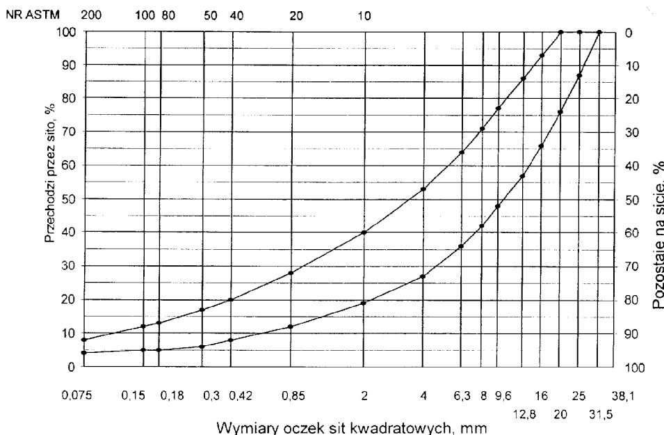
Rys. 1. Krzywe graniczne uziarnienia mieszanki mineralnej BA od 0 do 25mm do podbudowy nawierzchni drogi o obciążeniu ruchem KR 1 lub KR 2
