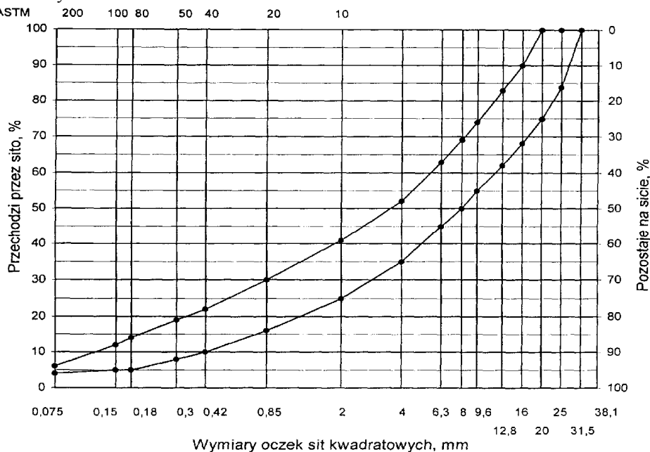
Rys. 5. Krzywe graniczne uziarnienia mieszanki mineralnej BA od 0 do 25 mm do warstwy wiążącej i wyrównawczej nawierzchni drogi o obciążeniu ruchem od KR3 do KR6
