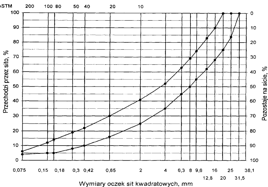
Rys. 6. Krzywe graniczne uziarnienia mieszanki mineralnej BA od 0 do 20 mm do warstwy wiążącej i wyrównawczej nawierzchni drogi o obciążeniu ruchem od KR3 do KR6
