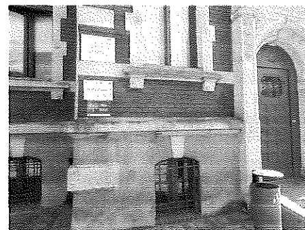
Zdjęcie nr 12: Hot Spot nr 5 – budynek Urzędu Miejskiego w Gubinie
