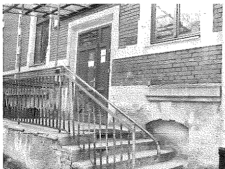
Zdjęcie nr 14: Hot Spot nr 5 - budynek Urzędu Miejskiego w Gubinie
